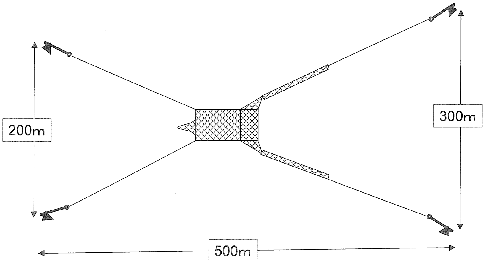
図 2 - 2 底建網の漁具概要 (平面図)
