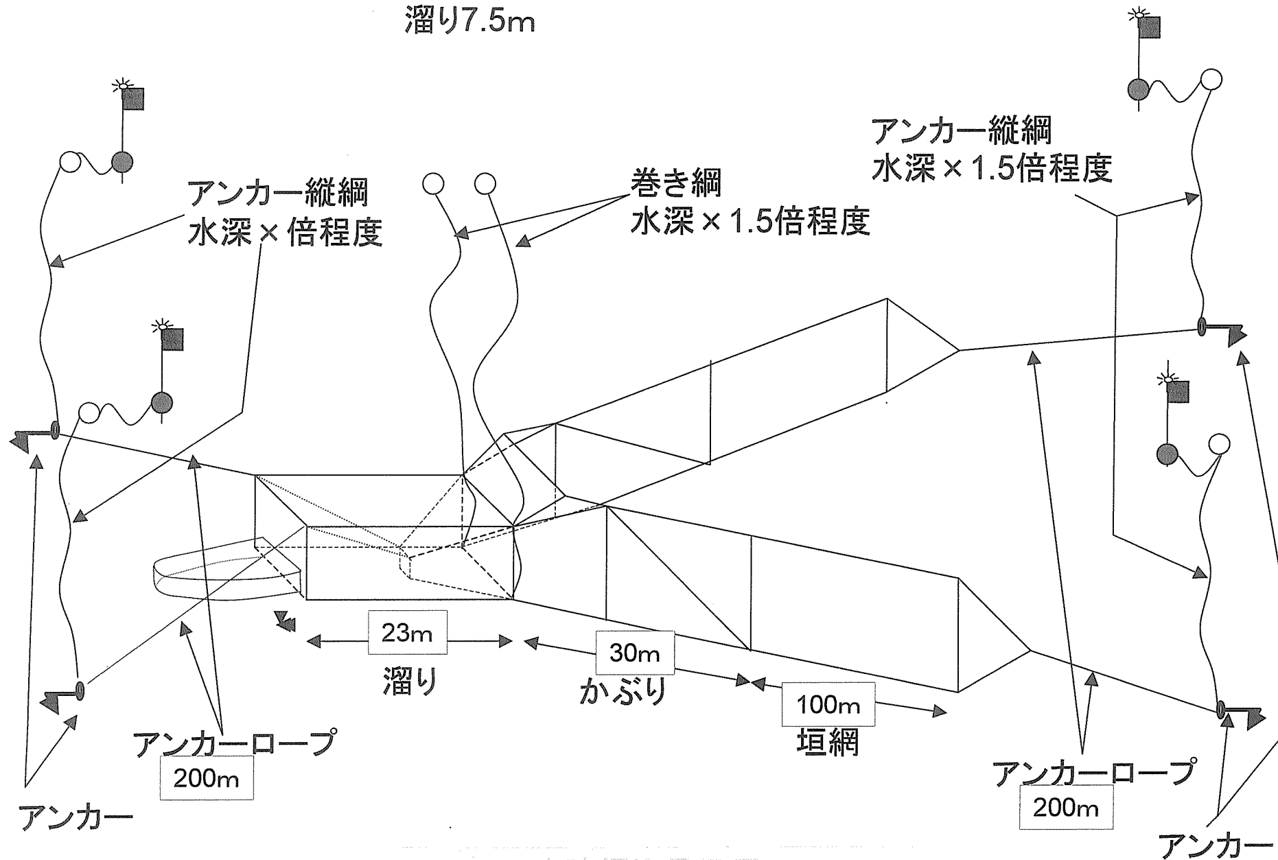
図2-1 底建網の漁具概要（鳥瞰図）
