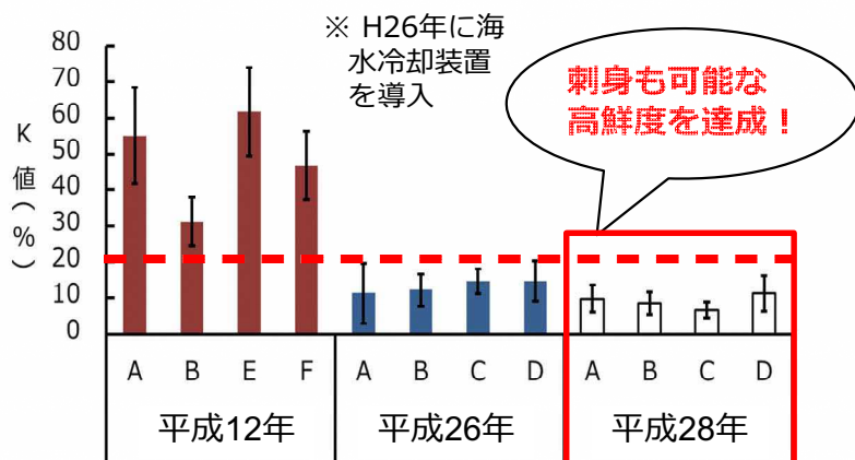
図2 海水冷却装置導入前後のミズガレイの K 値 (平均値) (A~F は船名)
