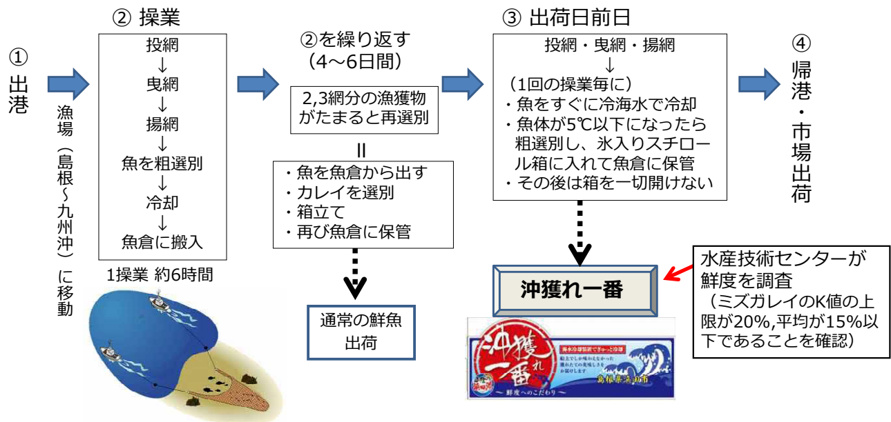
図3 沖合底びき網（2そうびき）の操業形態と漁獲物の処理手順
