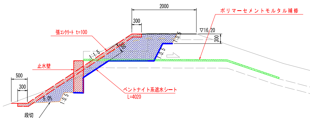
標準断面図
