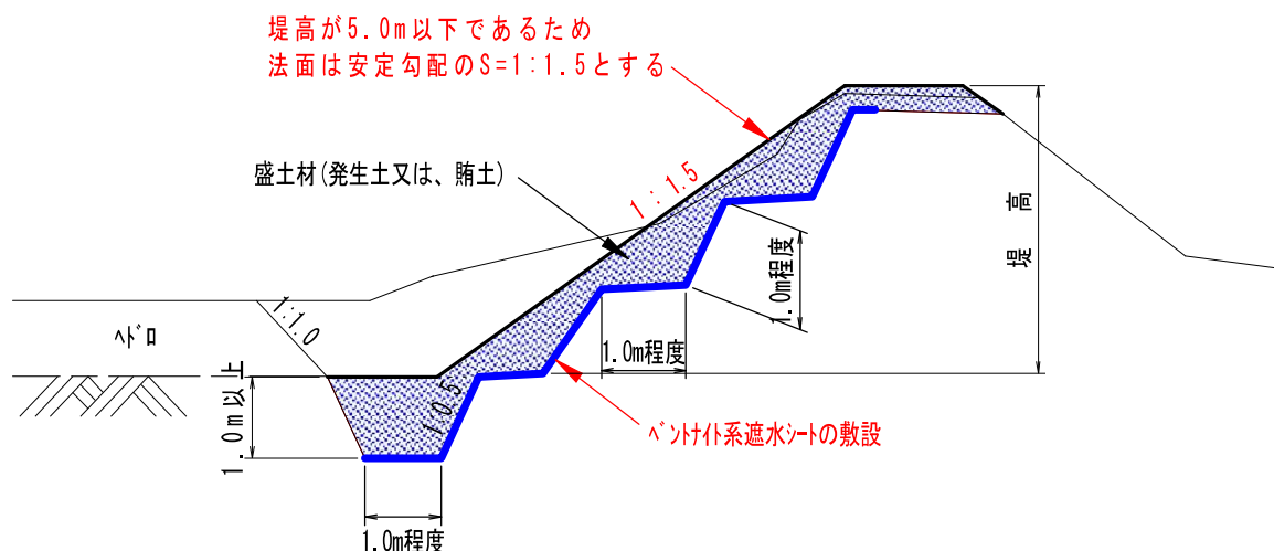
標準断面図
