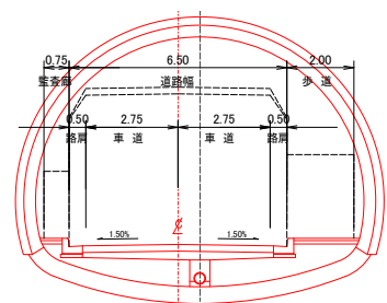
標準断面図
