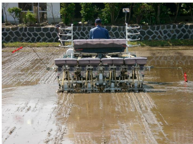
第12-4図 田植機装着播種機を使用した播種作業
