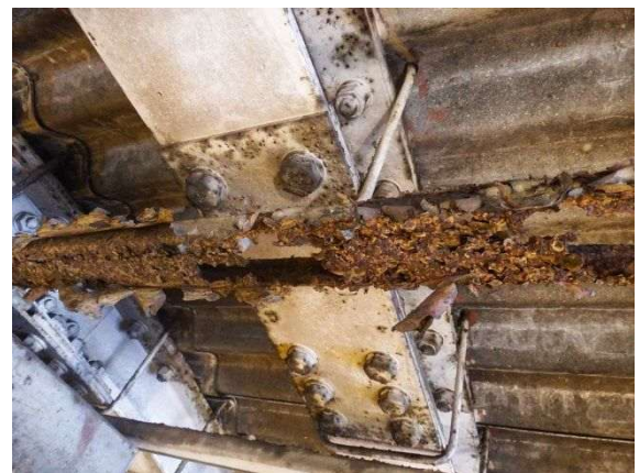
照明取付レールの断面欠損、破断
