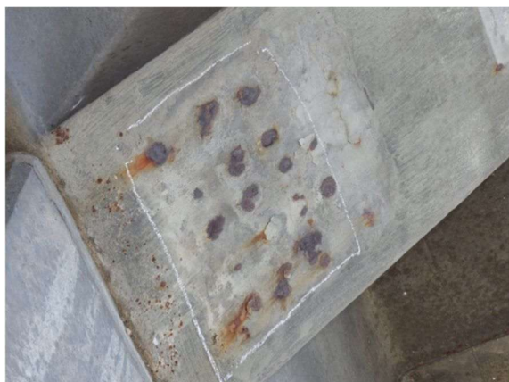
PC 鋼材からの錆汁（主梁）
