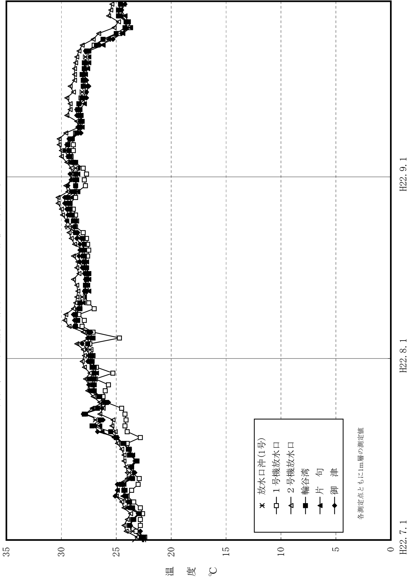
島根原子力発電所 沿岸定点の水温推移 (平成22年7月~9月)
