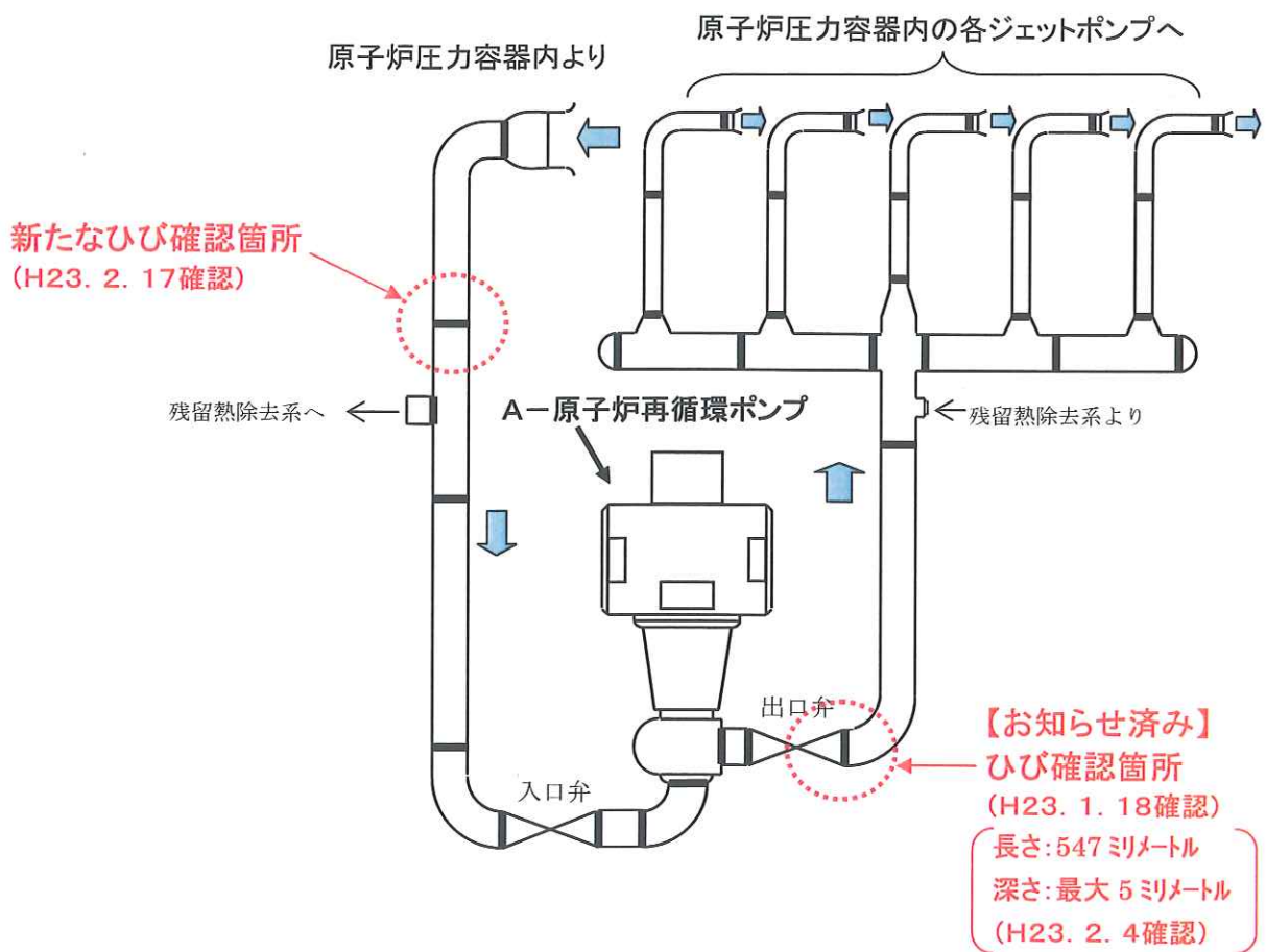
原子炉再循環系配管系統概略図 (ひび確認箇所)
