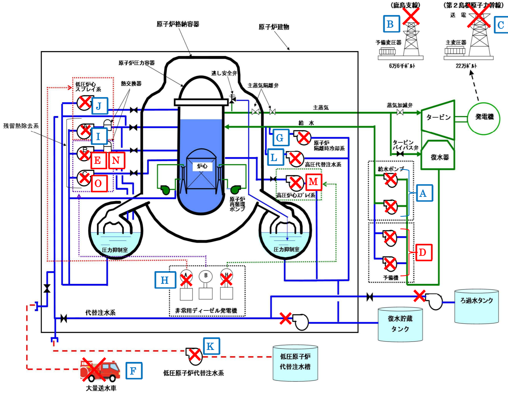
【島根原子力発電所2号機 事象想定図】
