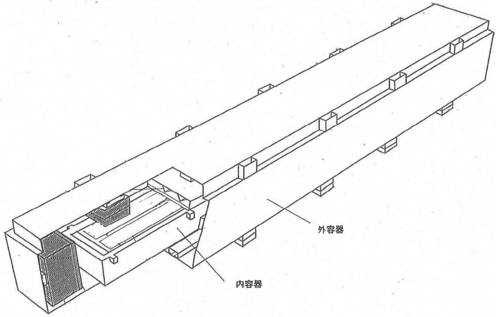
輸送容器概観図 (NT-IV型)
