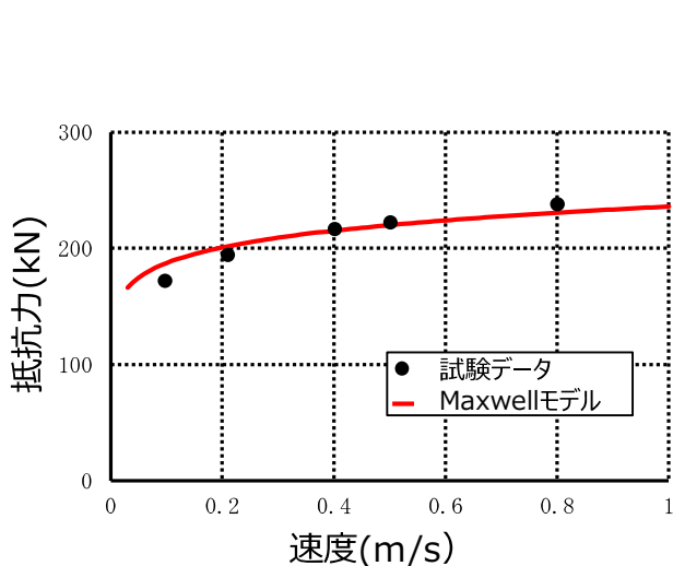
速度と抵抗力の関係
