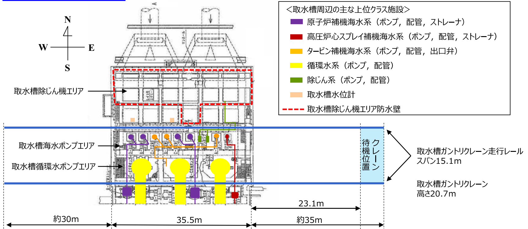
取水槽ガントリクレーンの設置位置及び取水槽周辺の上位クラス施設概要
