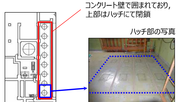
図3 復水ろ過脱塩器室
