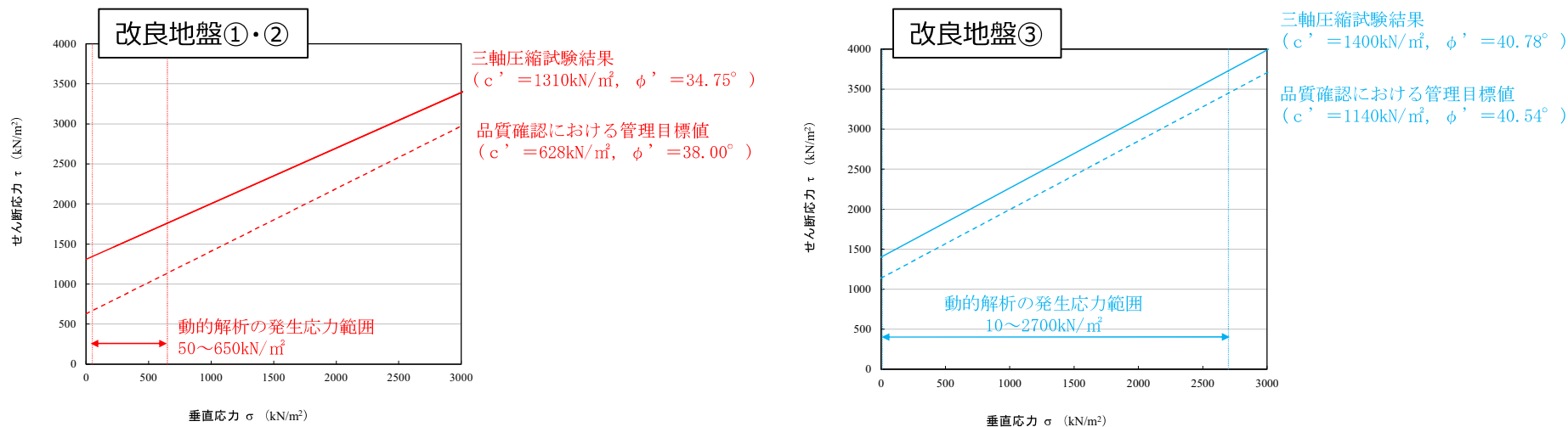
図3 三軸圧縮試験結果
