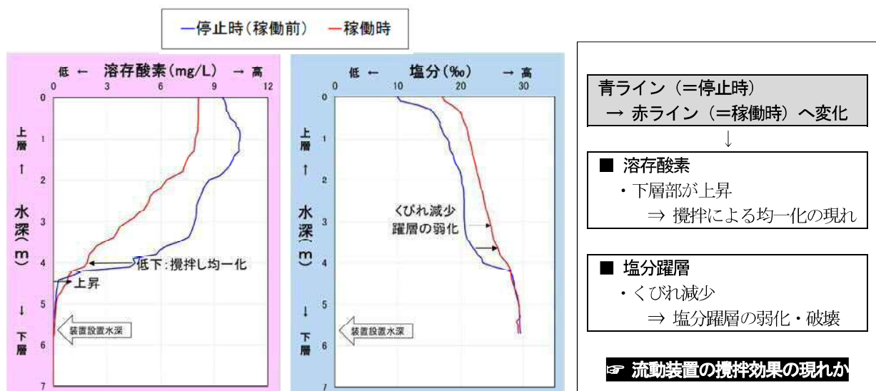
200m離れた地点の鉛直分布(溶存酸素・塩分)
