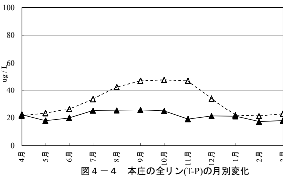
図 4-4 本庄の全リン(T-P)の月別変化
