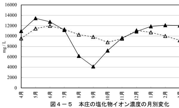
図 4-5 本庄の塩化物イオン濃度の月別変化
