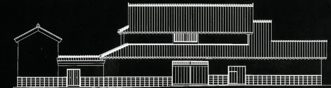
上：重要文化財熊谷家住宅復元図 下：同住宅正面図
