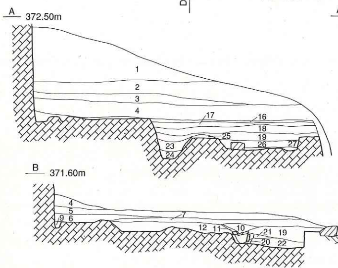
第2図 岩盤加工遺構 第2段 平面図・断面図 (S=1/60) ※一部改変
