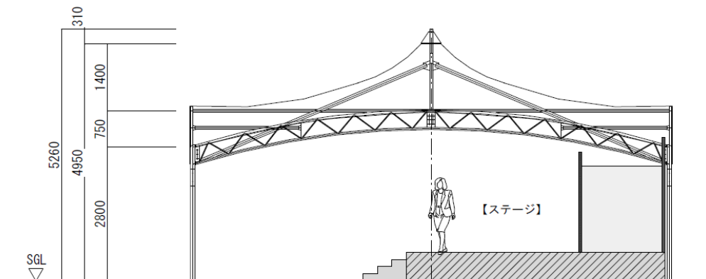
○側面立面図
