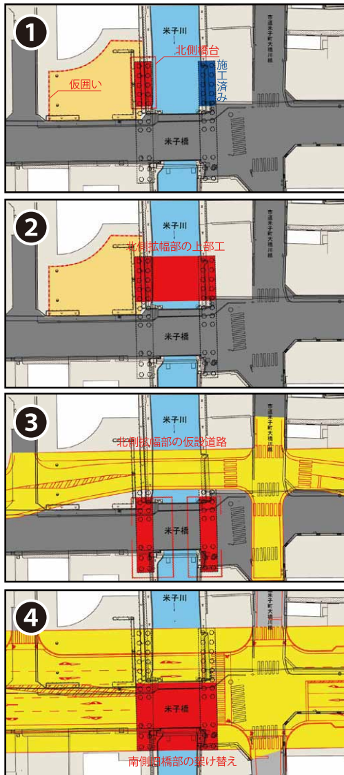
※上記は、米子橋整備イメージです。親柱・高欄のデザイン及び各施設配置は、検討中です。
