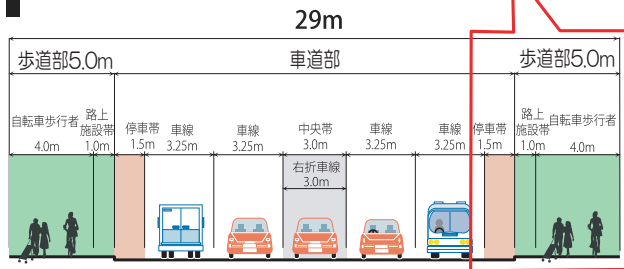
標準断面図(幅員29m)
