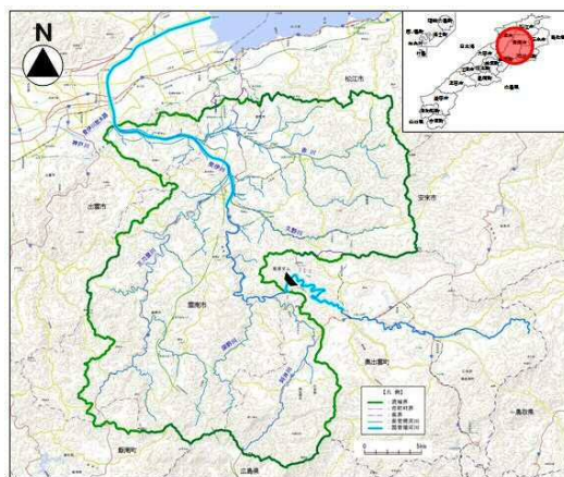
斐伊川水系中流支川域流域図
