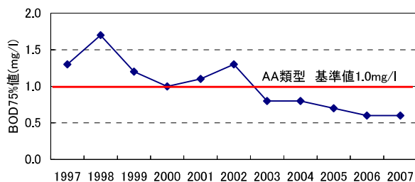
図 3-3(1) 祝原地点のBOD75%値の経年変化
