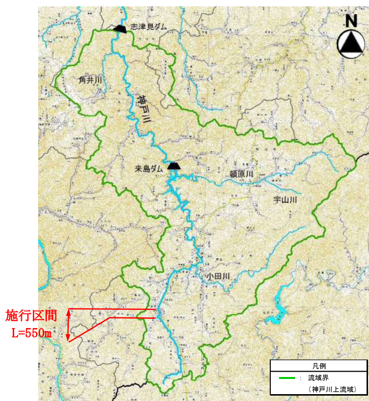
図 4-1 施行位置図
