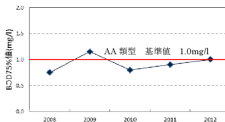
図 3-3(2) 潮橋地点のBOD75%値の経年変化
