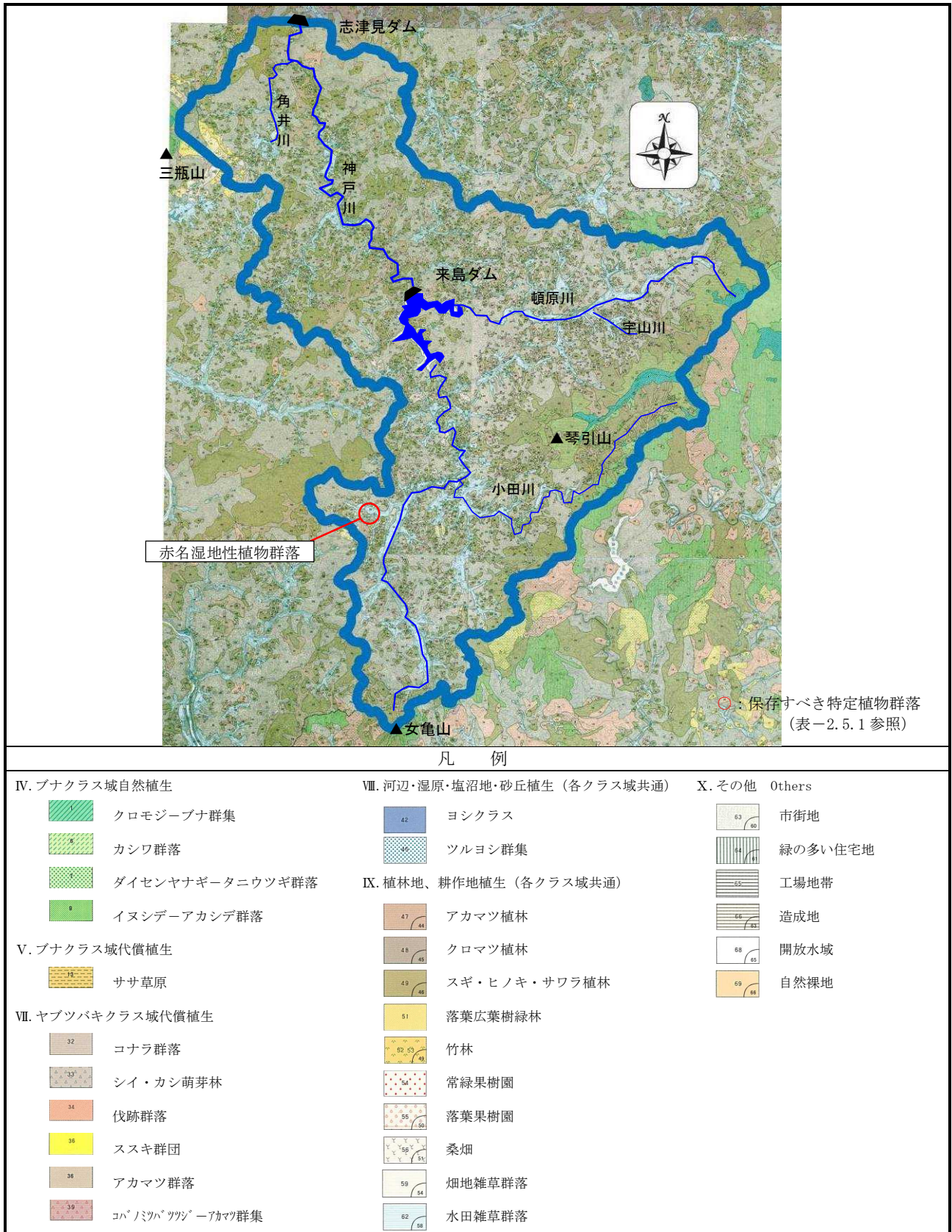
図-2.4.1 現存植生図
