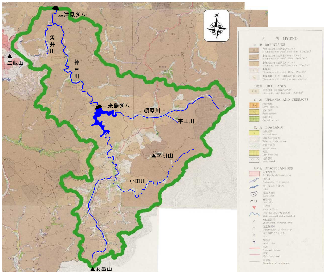
図一 2.1.1 地形分類図
