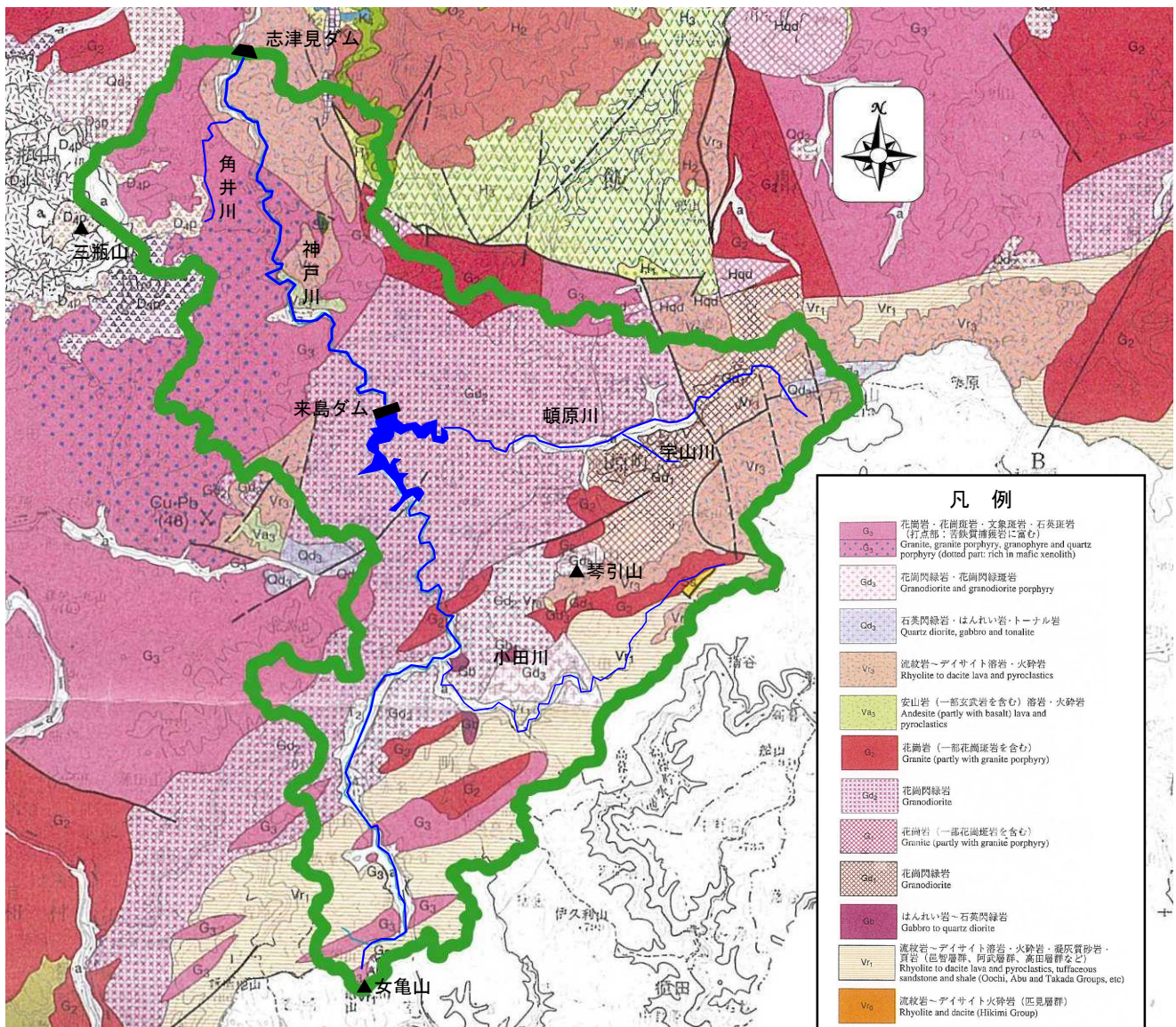
図-2.2.1 地質図 (S=1/200,000)
