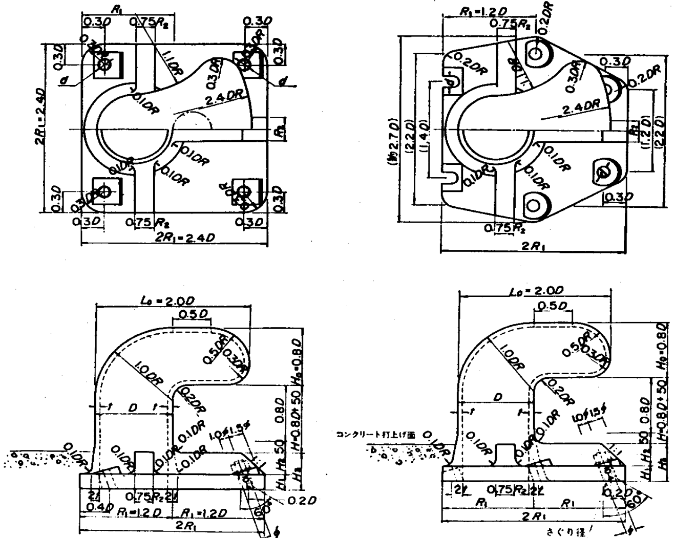
設計けん引力が50,100,150,250 kNの場合
