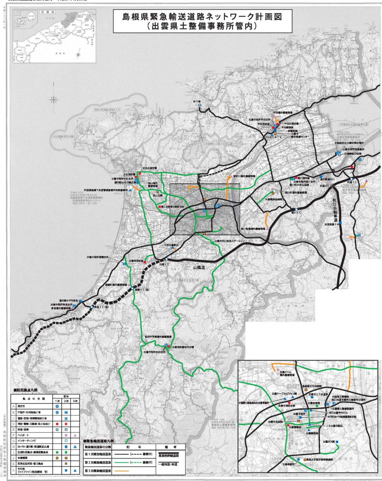
図 2-26 緊急輸送道路網図（出雲県土整備事務所管内 平成 25 年 6 月 1 日時点）
