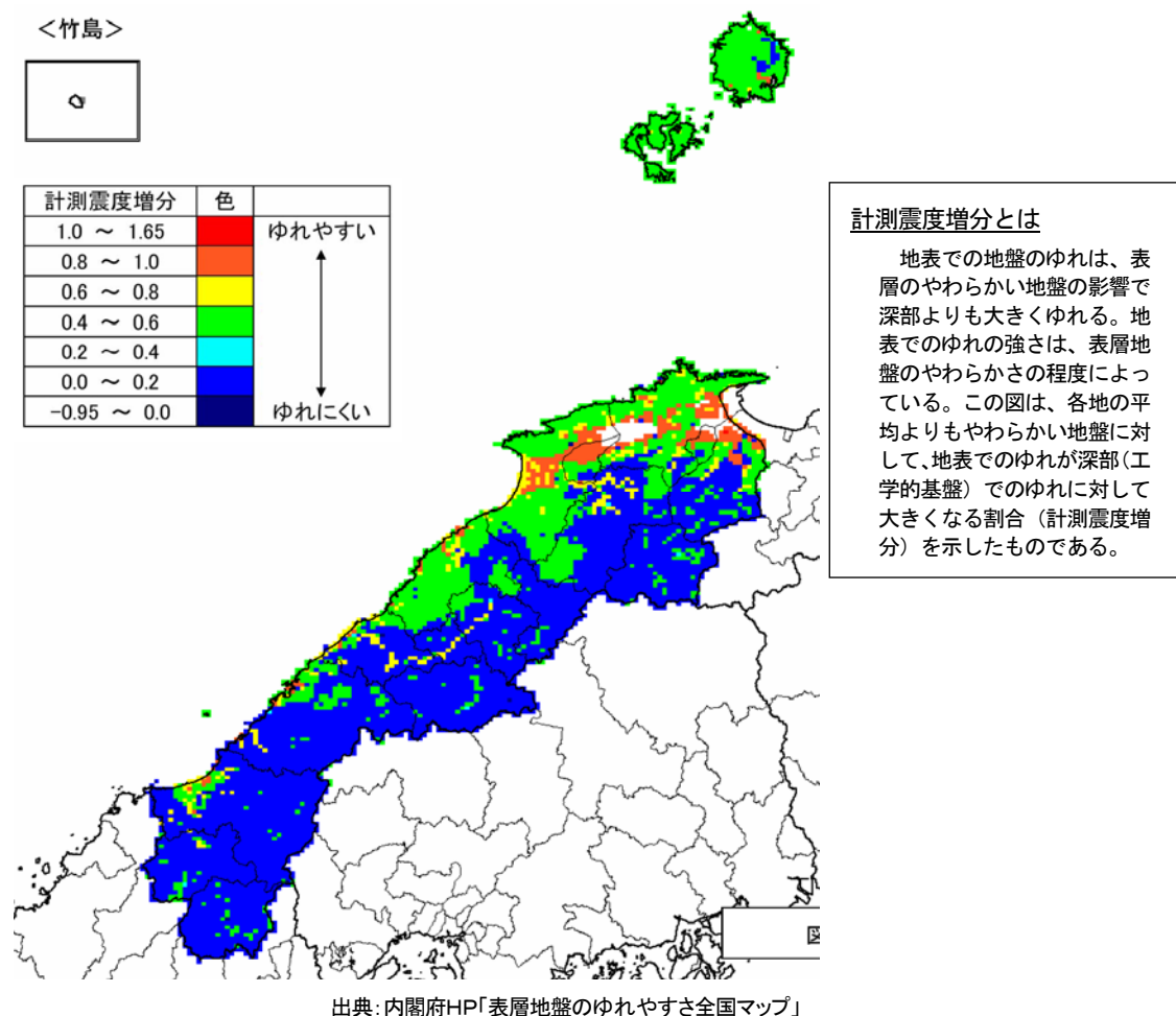
図 2-4 表層地盤のゆれやすさ（島根県）
