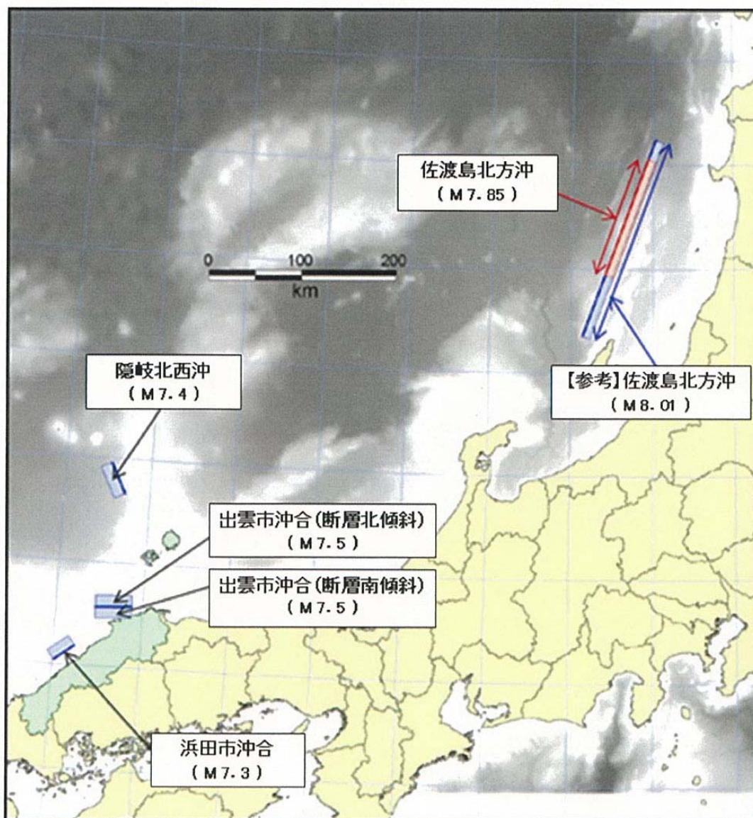
図 2-2 各地震における震度分布
