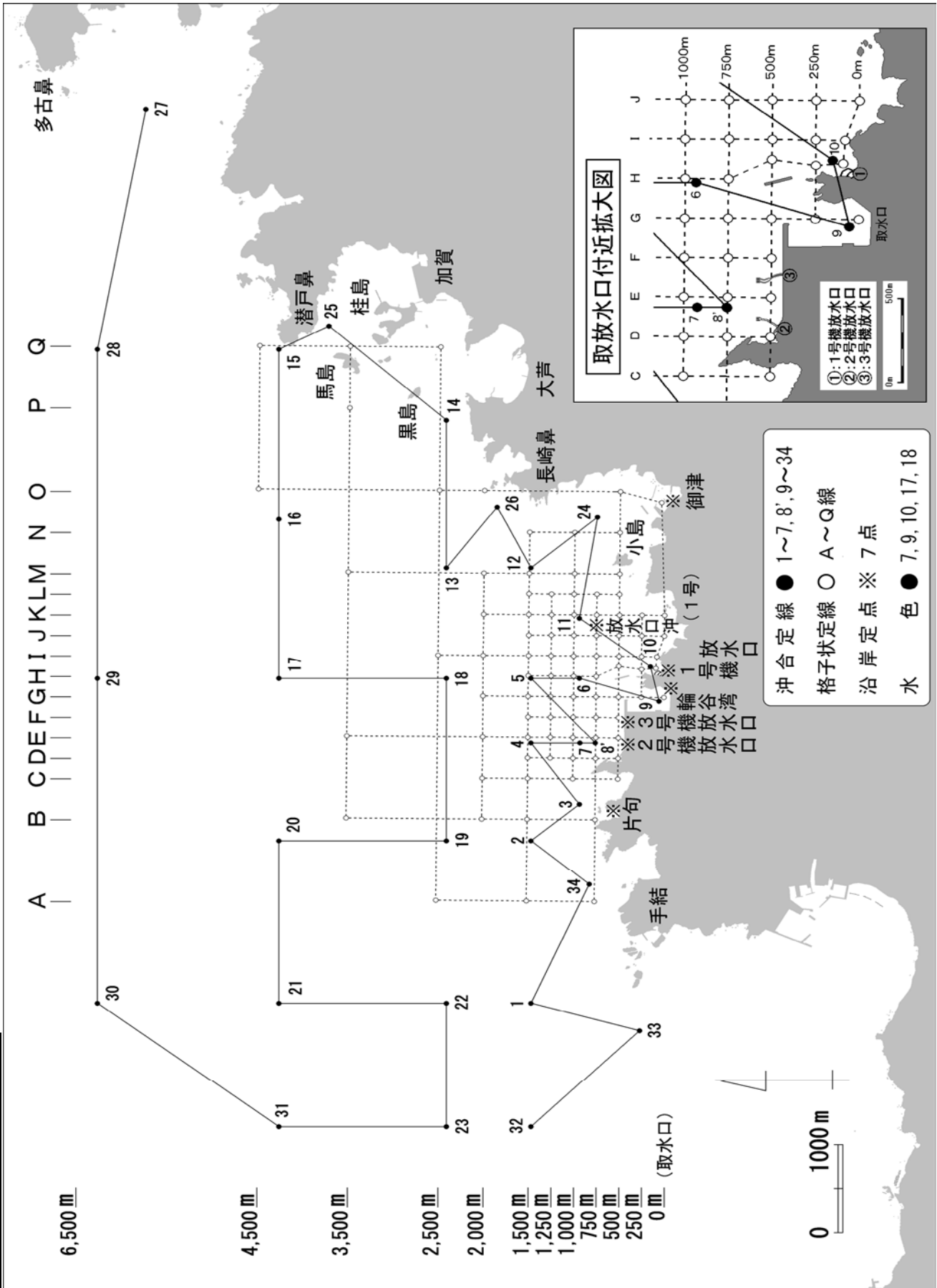
温排水測定定点図
