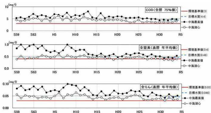
中海の水質の経年変化
